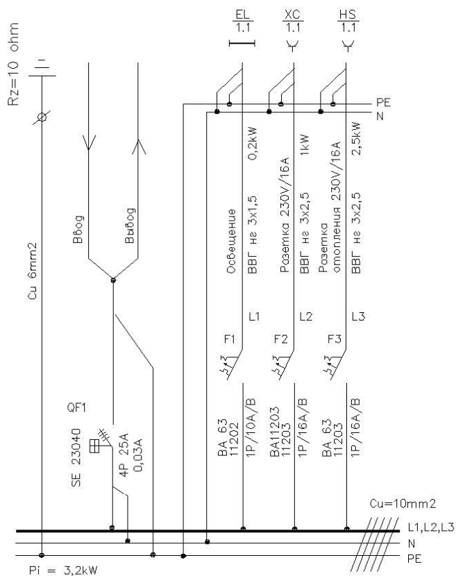
Щит распределительный UV1
