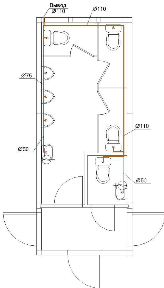
Схема канализации
