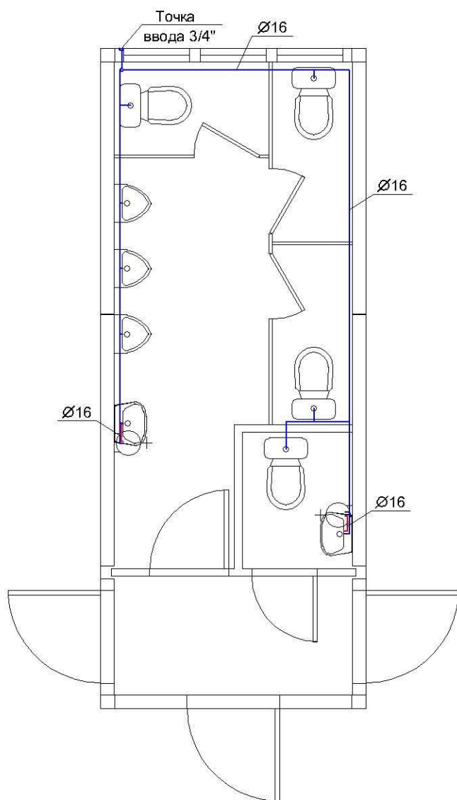
Схема водопровода
