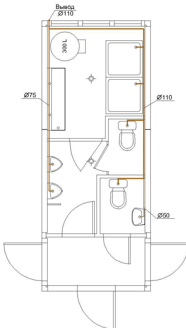
Схема канализации
