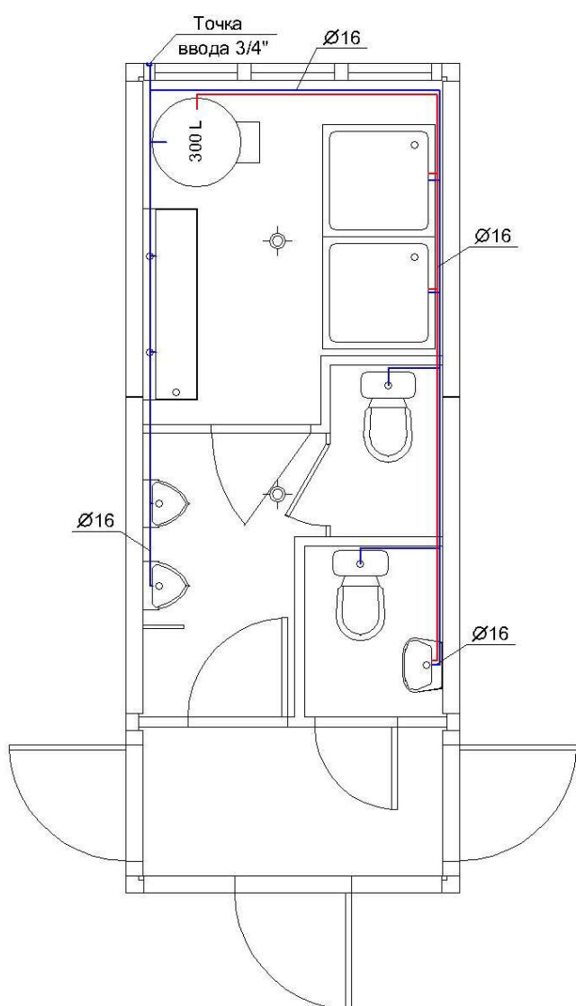
Схема водопровода
